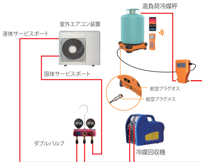
冷媒回収の見取り図
